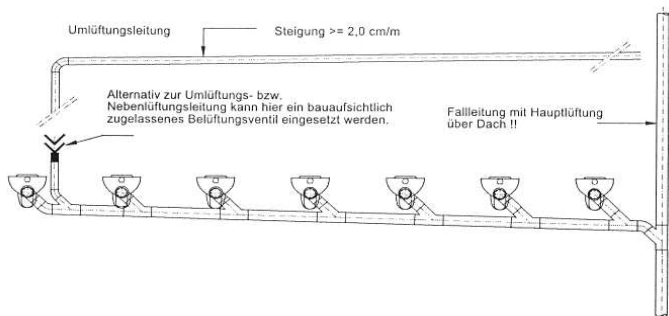
Abb 2: Ersatz einer Neben- bzw. Umlüftungsleitung durch Belüftungsventil bei einer hochbelasteten Sammelanschlußleitung
